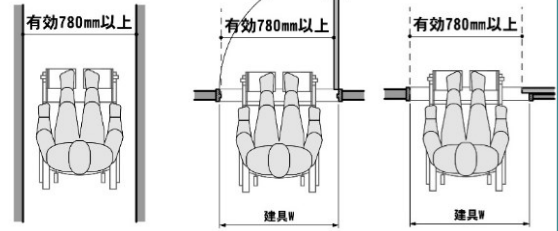
通路の有効幅員 出入口の有効幅員
